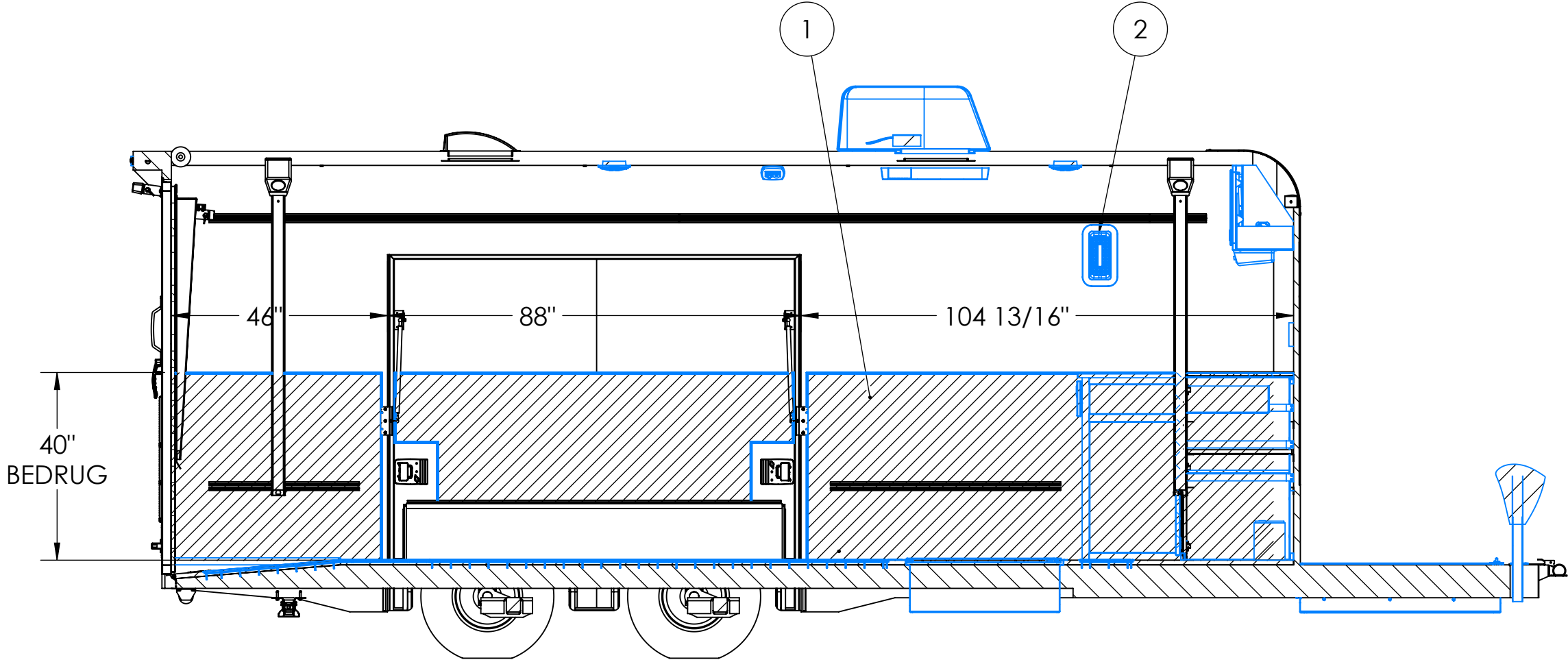
SECTION D-D
